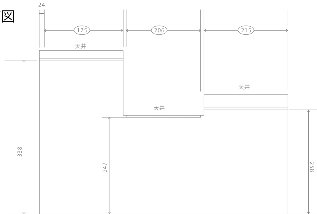
西側立面図
